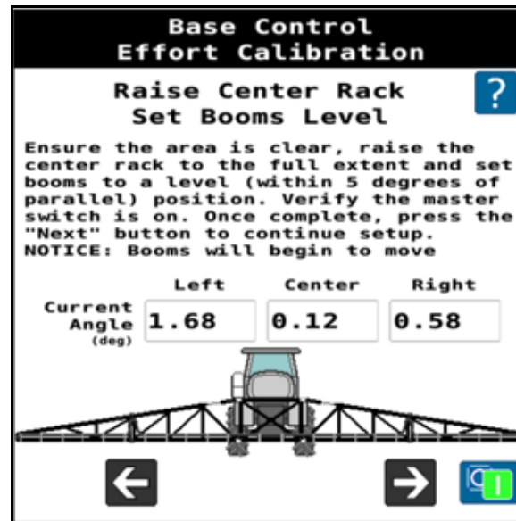
FIGURA 14. Calibración del esfuerzo de control de base
