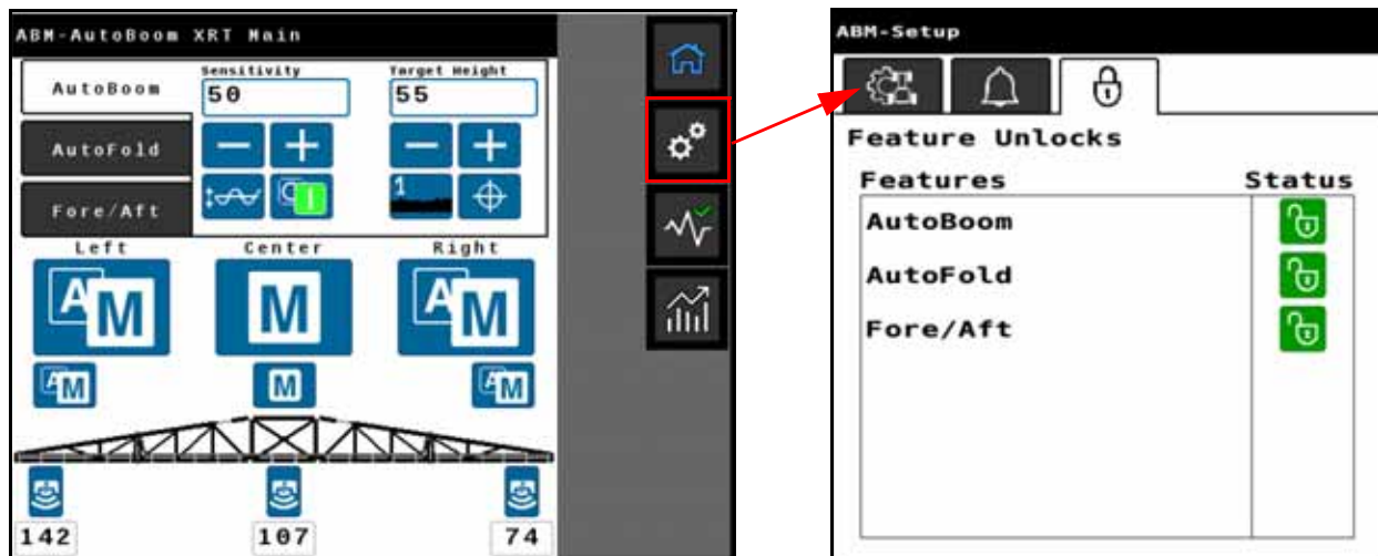
FIGURA 39. Pantalla de desbloqueo de funciones
