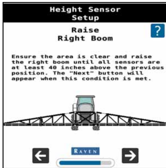
FIGURA 13. Configuración de sensor de altura: elevado de pluma derecha
