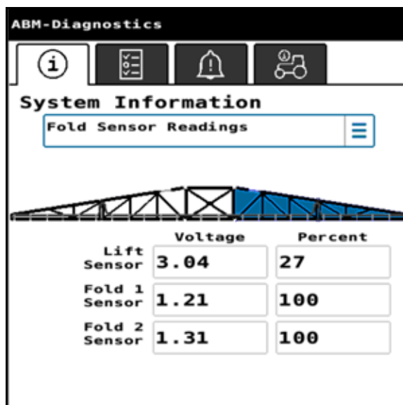
FIGURA 7. Lecturas del sensor de plegado
