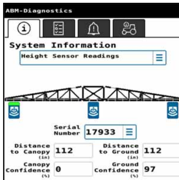
FIGURA 11. Lectura del sensor de altura
