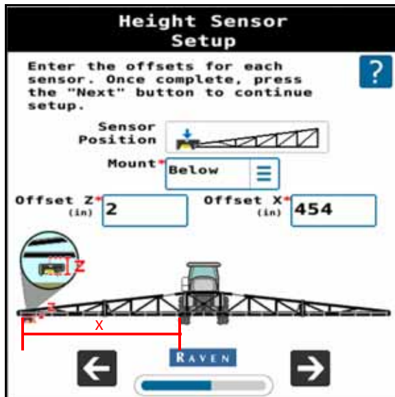
FIGURA 10. Configuración de sensor de altura
