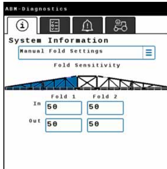
FIGURA 2. Configuraciones del plegado de la máquina
