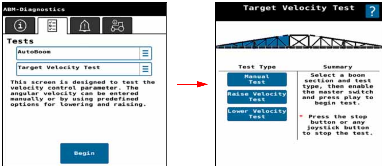
FIGURA 18. Prueba de velocidad objetivo
