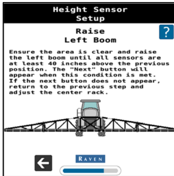
FIGURA 19. Configuración de sensor de altura: elevación de pluma izquierda
