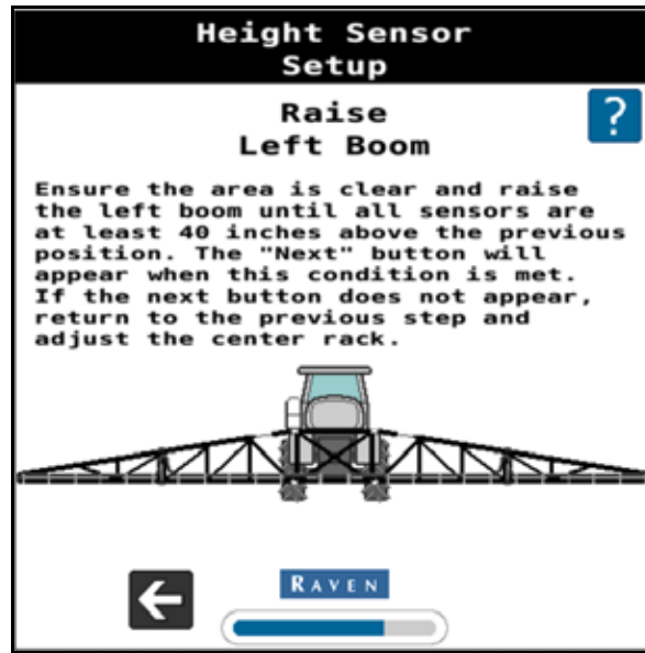
FIGURA 12. Configuración de sensor de altura: elevado de pluma izquierda
