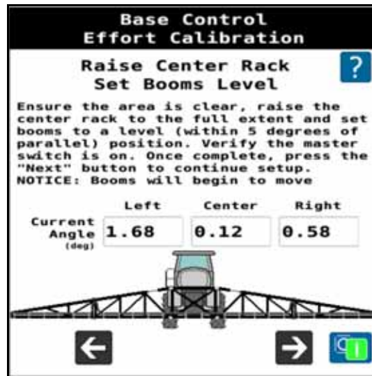
FIGURA 22. Calibración del esfuerzo de control de base
