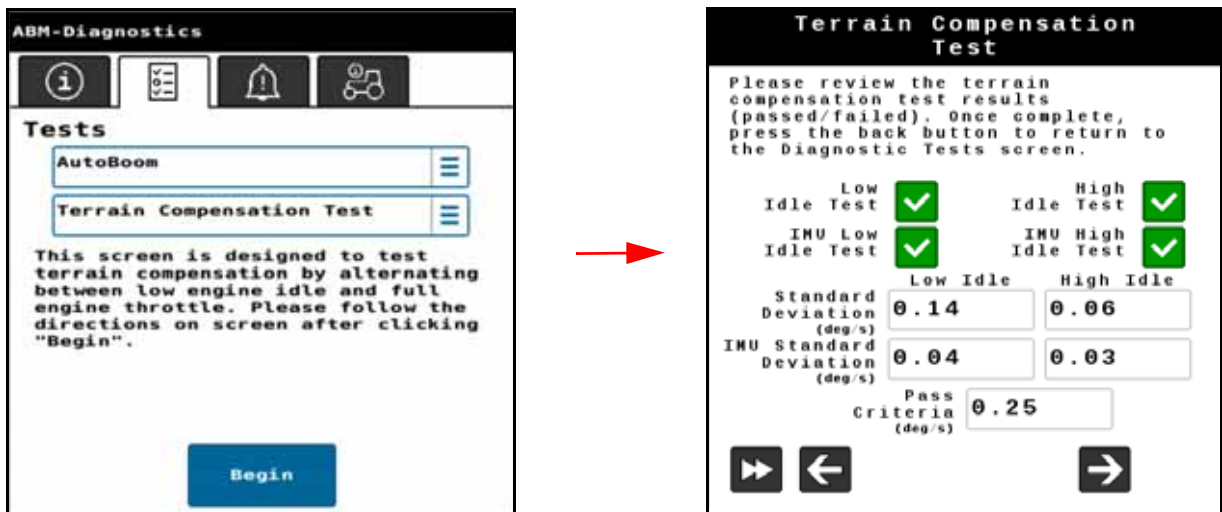
FIGURA 21. Prueba de compensación del terreno
