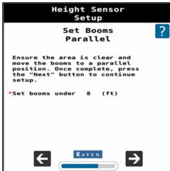
FIGURA 11. Configuración de sensor de altura: colocación paralela de plumas
