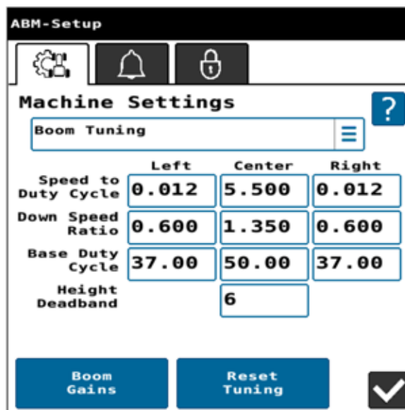
FIGURA 15. Pantallas de ajuste fino de la pluma
