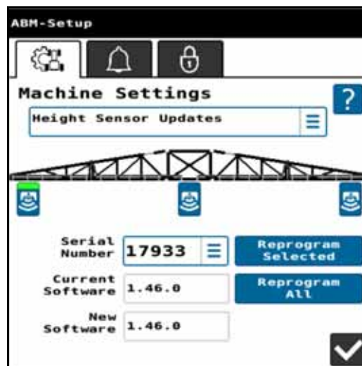
FIGURA 11. Actualizaciones del sensor de altura
