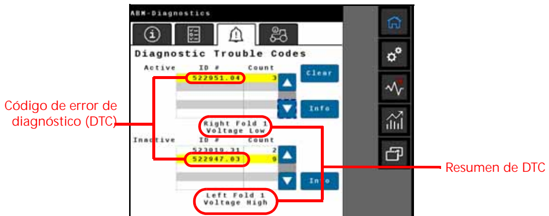
FIGURA 25. Pantalla de códigos de error de diagnóstico
