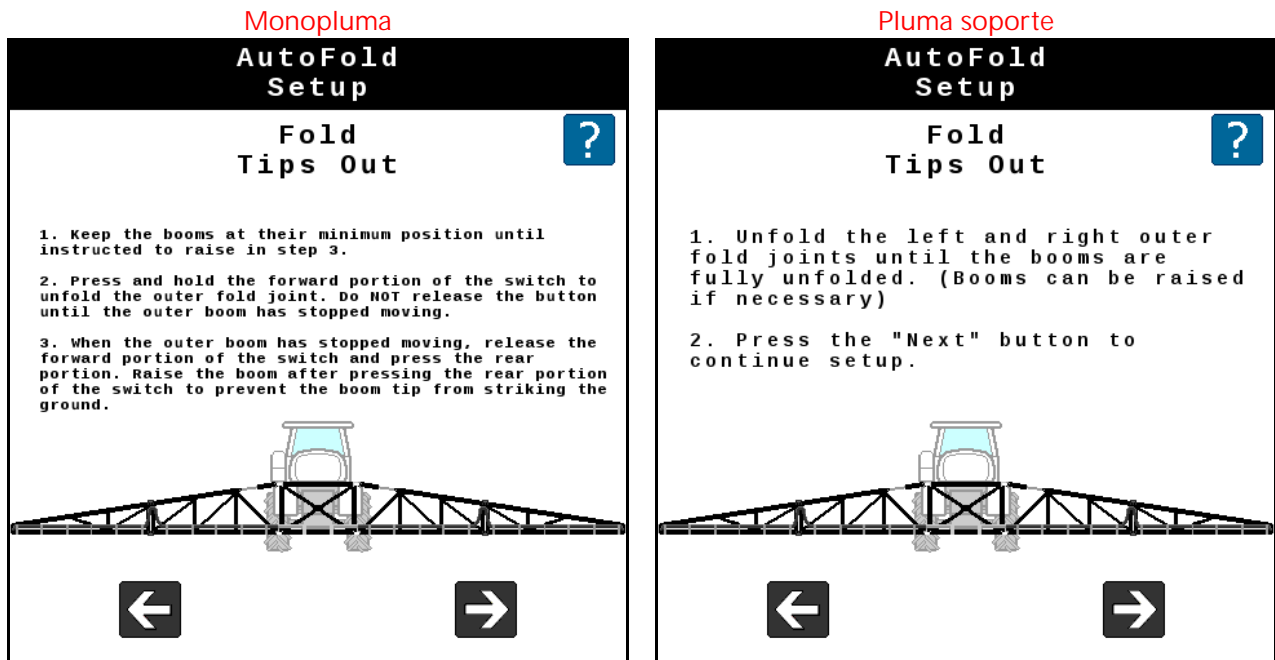
FIGURA 31. Desplegar puntas hacia afuera
