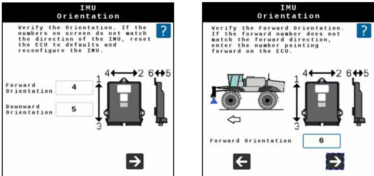
FIGURA 8. Orientación de la IMU
