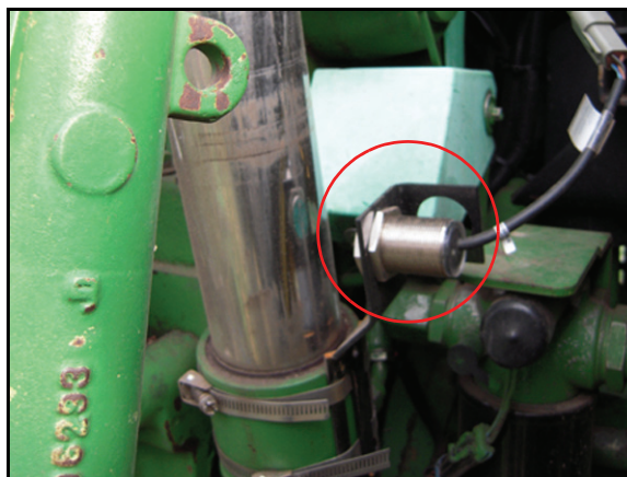
Монтаж выключателя для сеялки с трехточечным креплением
