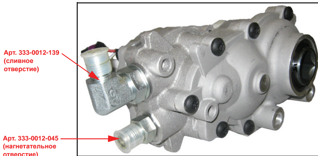
FIGURE 5. Фитинги, установленные на гидравлические двигатели
