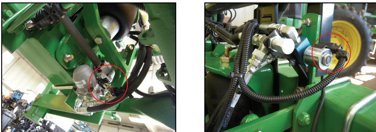
FIGURE 4. Подключения соединительного кабеля на модулях рядков
