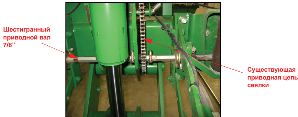
FIGURE 2. Существующий шестигранный вал машины
