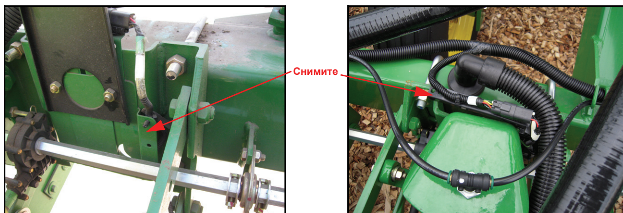
FIGURE 7. Кабельные держатели
