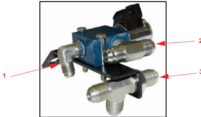
FIGURE 11. Узел ШИМ-клапана для средних модулей рядков
