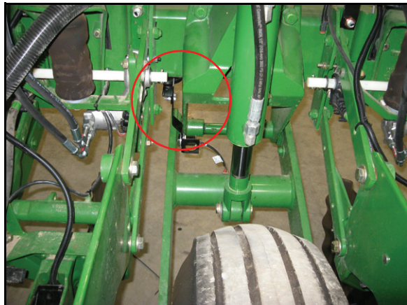
Монтаж переключателя для прицепной сеялки
