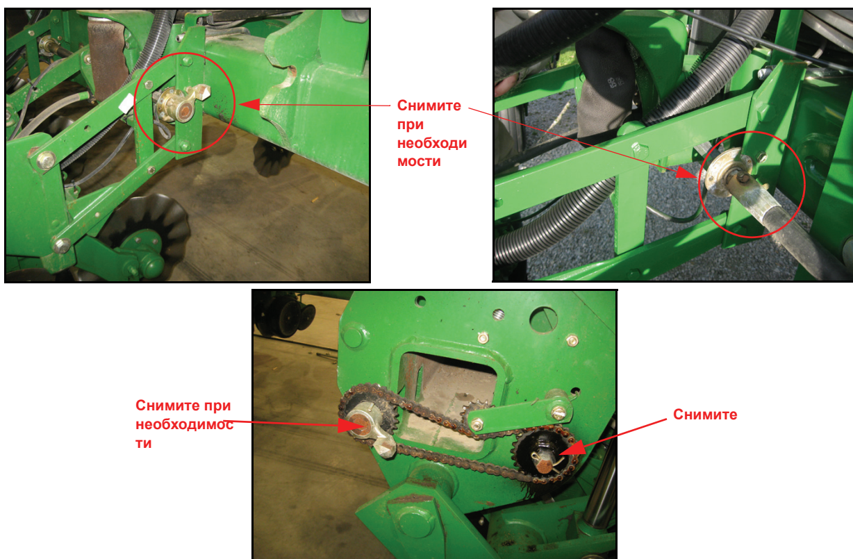
FIGURE 3. Дополнительные опорные подшипники машины
