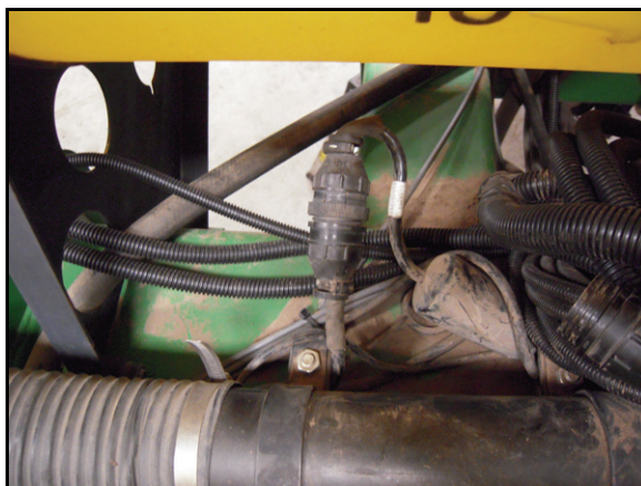
FIGURE 2. Подключение датчика семяпровода
