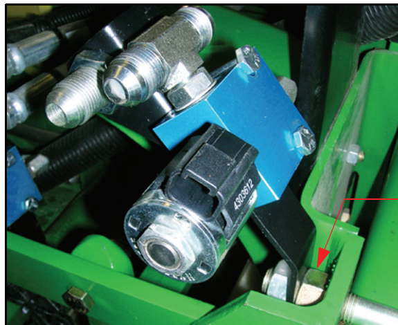
FIGURE 12. Установленный ШИМ-клапан
