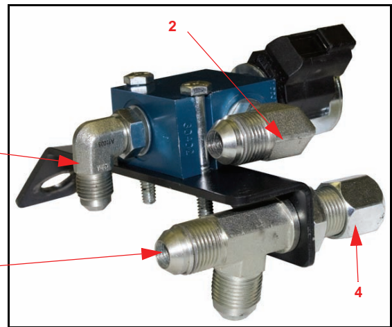
Правый ШИМ-клапан в сборе
